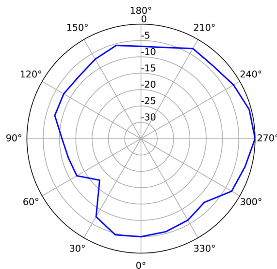
5G (Vertical)
