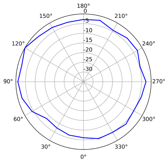
2.4G (Vertical)
