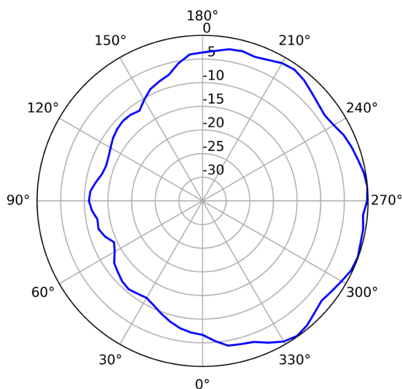
5G (Horizontal)
