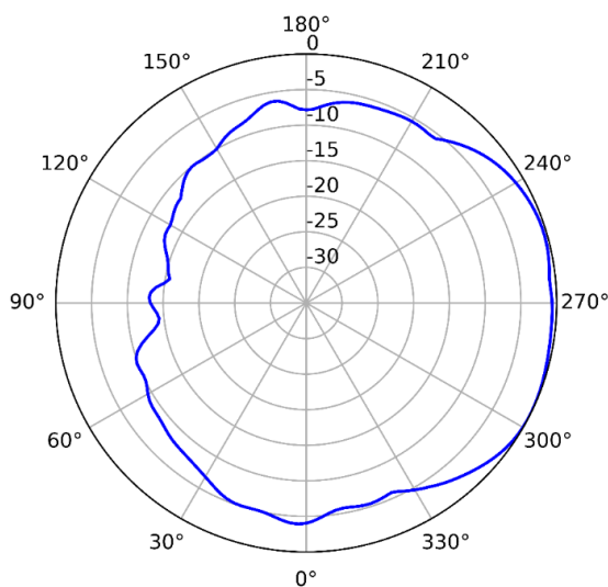
5GHz (Horizontal)
