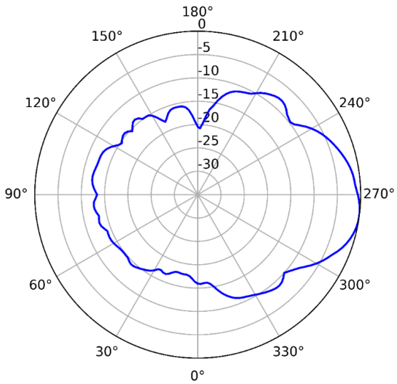
2.4GHz (Vertical)
