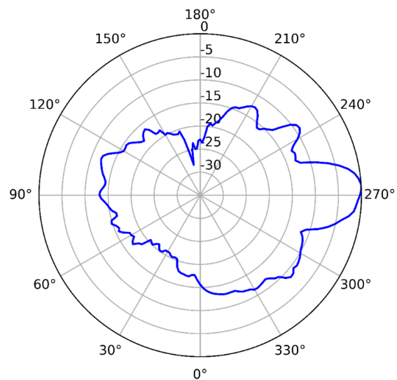
5GHz (Vertical)
