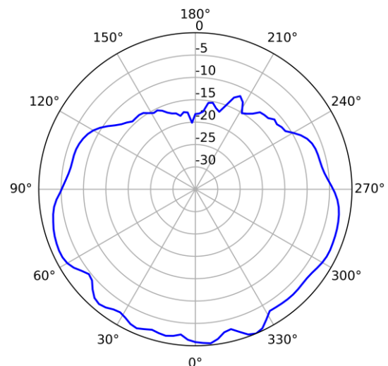
5GHz (Vertical)
