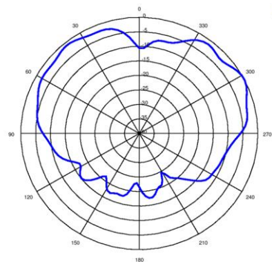
5G-2(PHI=90)
