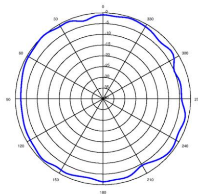
5G-2(PHI=0)
