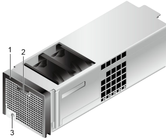
Figure 4-44 Fan module
