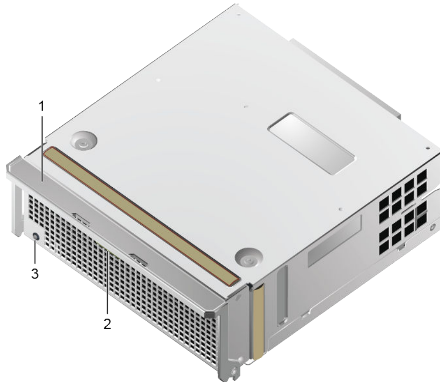
Figure 4-57 Fan module
